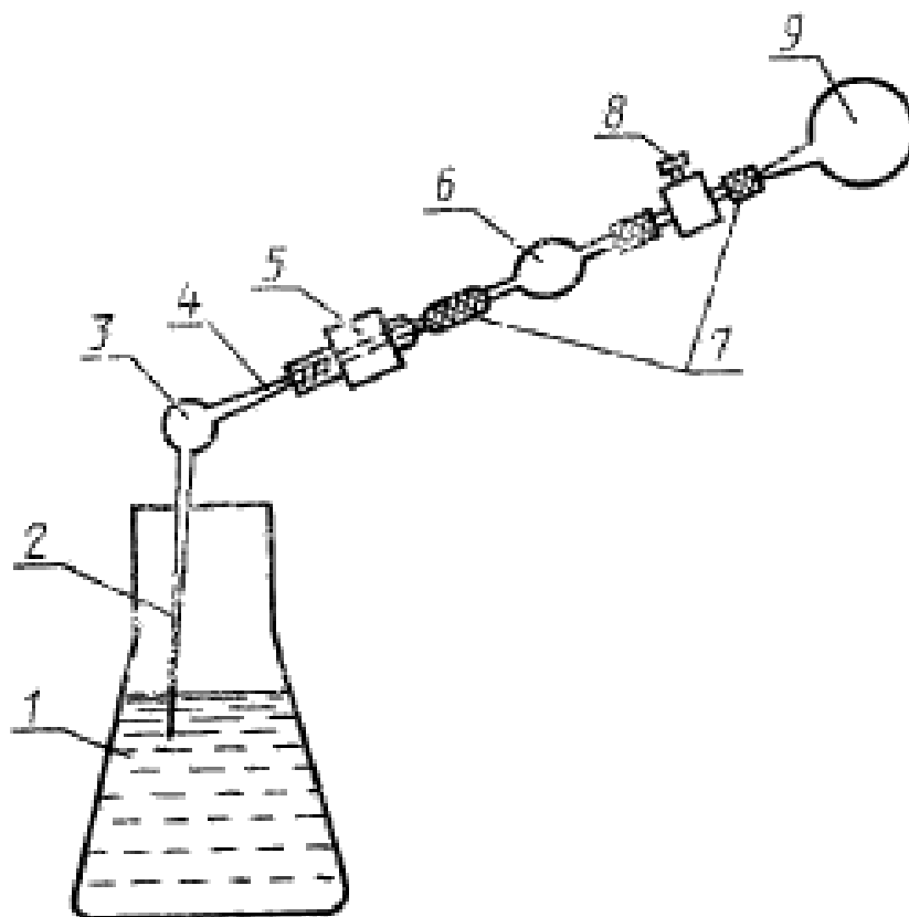
1—колба с меланжем; 2, 4—капиллярные концы ампулы; 3—ампула; 5—фторопластовый муфта; 6—стеклянный индикатор; 7—гибкий шланг; 8—вентиль; 9—резиновая груша
